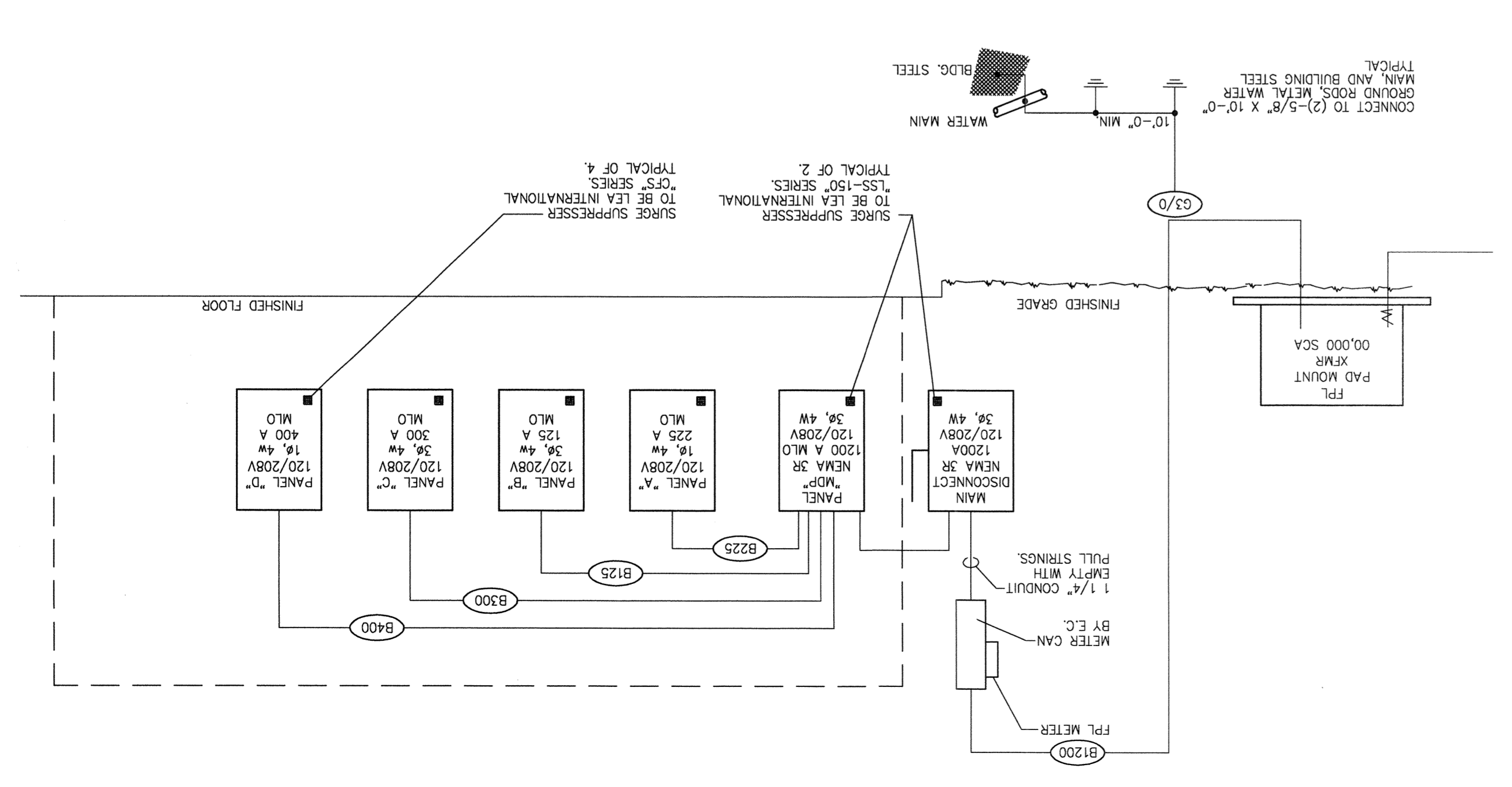
ELECTRICAL RISER SCALE: NONE
